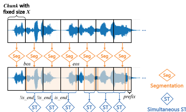
図 1: ストリーミング同時音声翻訳システムの概要
