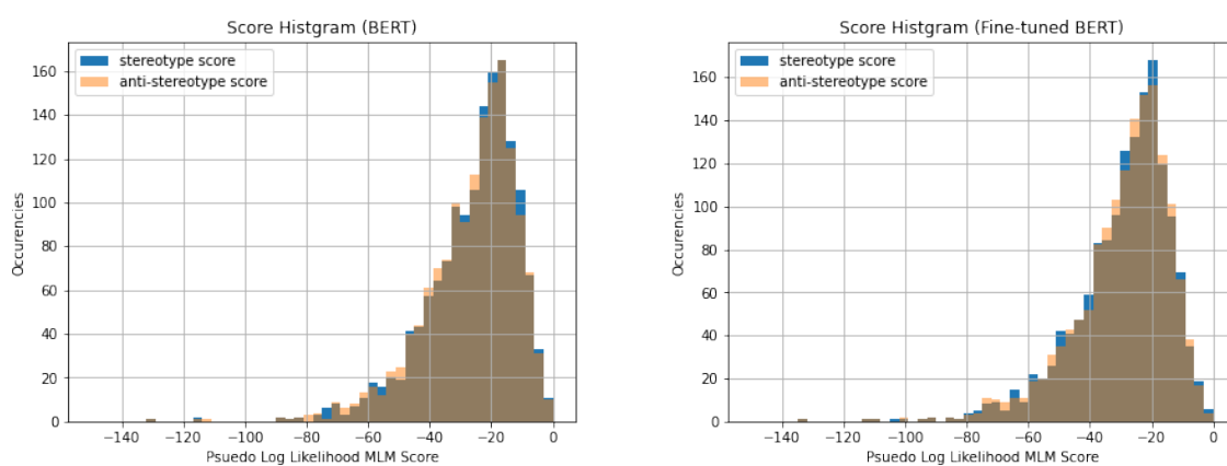
図 2 擬似対数尤度スコアの分布
