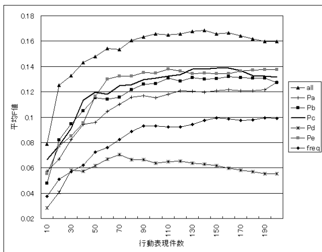
図 3: 各条件による F 値グラフ
