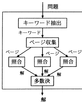
図1 汎用的解法の概要
