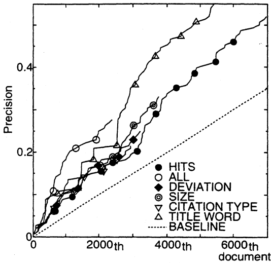
図 1: 上位 n 論文の精度の比較
